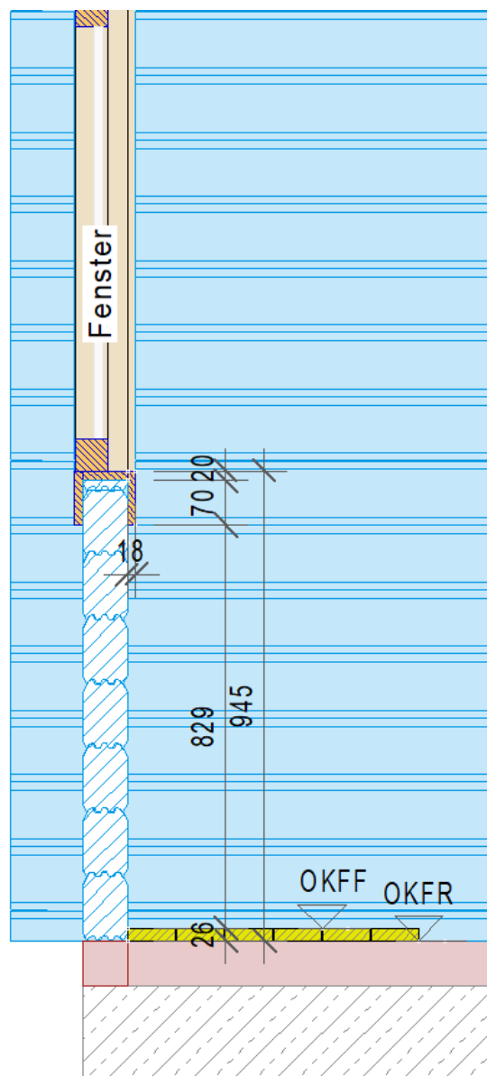
Abbildung 1 Beispielzeichnung (die Höhen können auf den Wohnhausstandard adaptiert werden)
